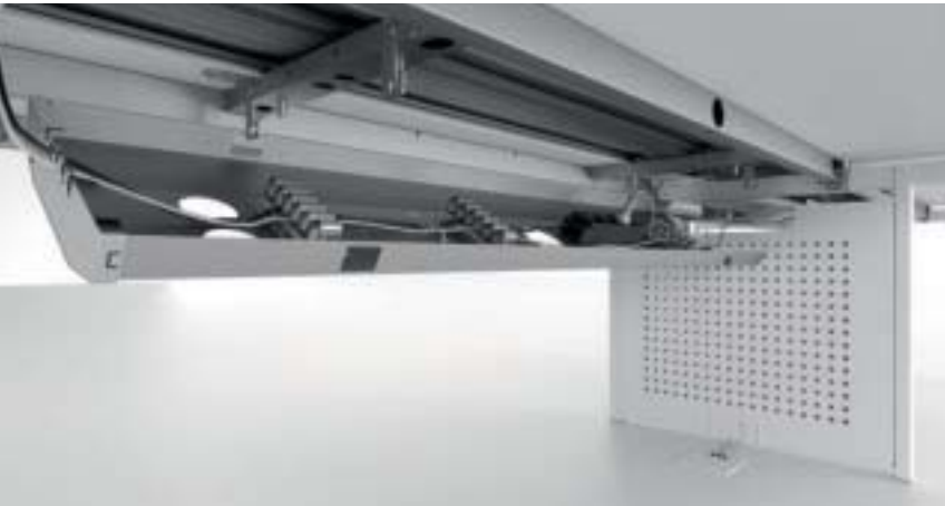
Dettaglio ispezione canale passacavi - Detail inspection cable channel
